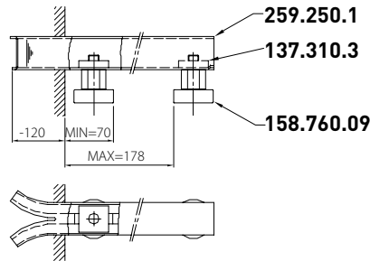
259.250/1 (inclusief draagstukken 137.310.3)
