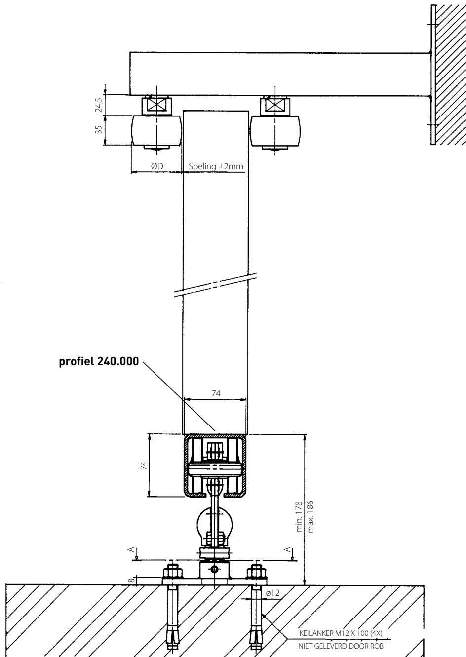
Doorsnede A-A
