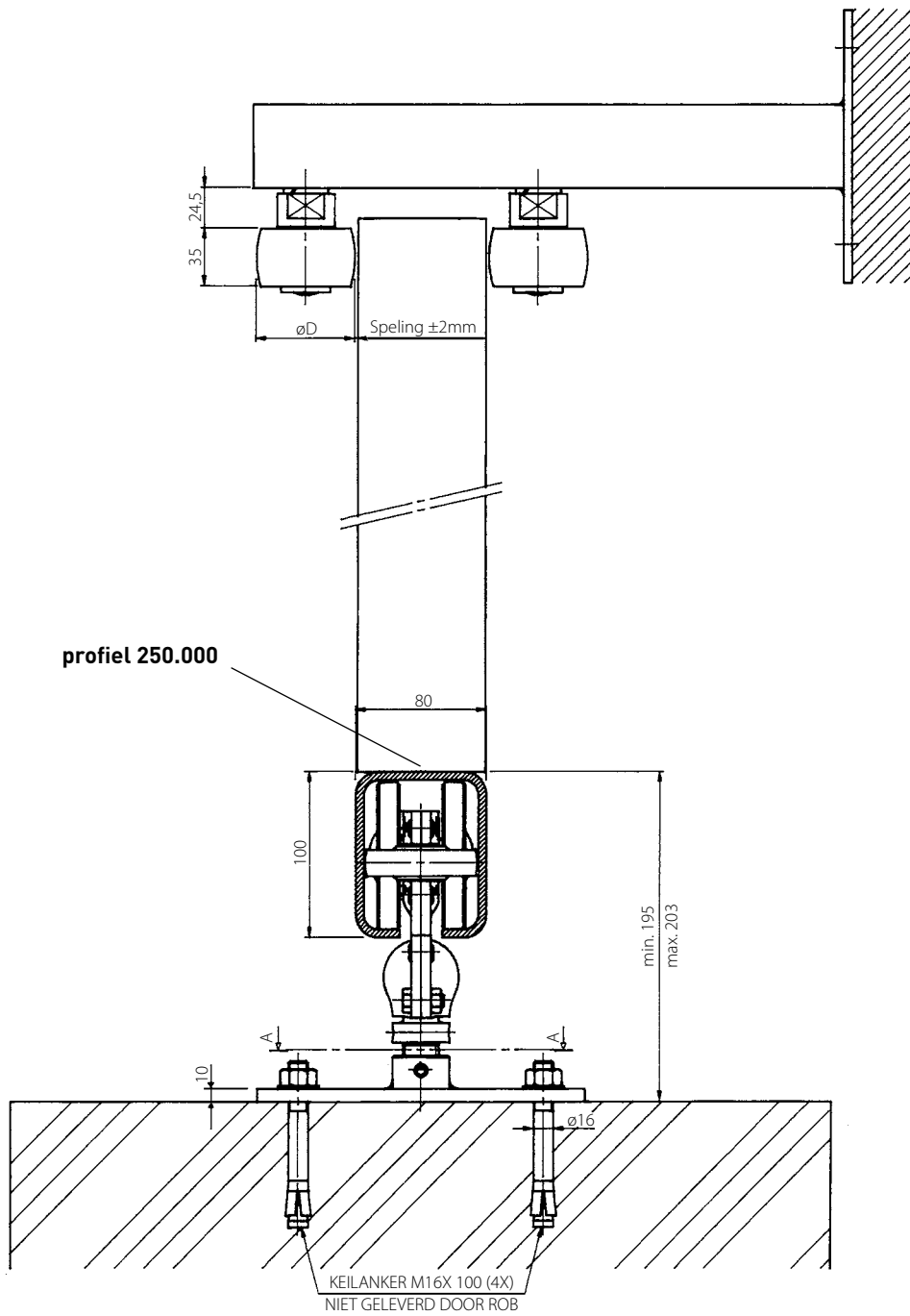
doorsnede A-A
