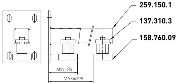
259.150/1 (inclusief draagstukken 137.310.3)
