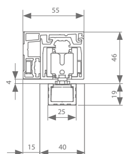
Fijación vista a pared 40 mm
