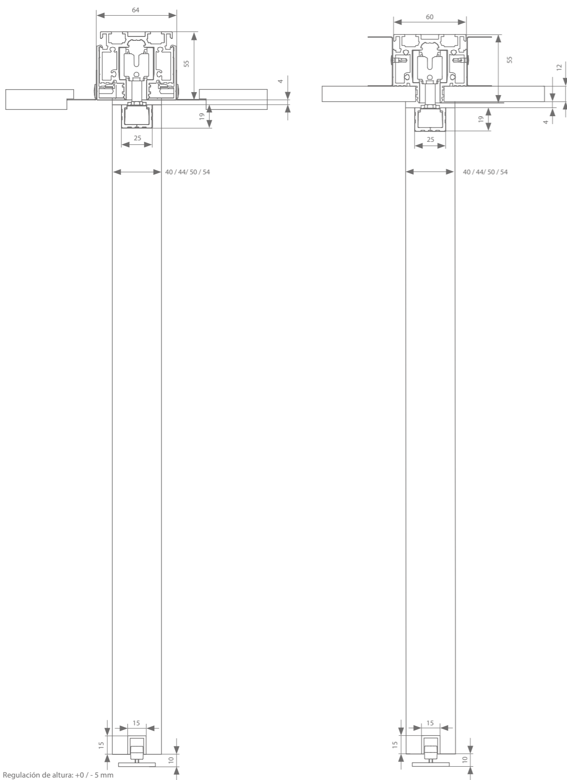
Para falsos techos técnicos (1+2)
