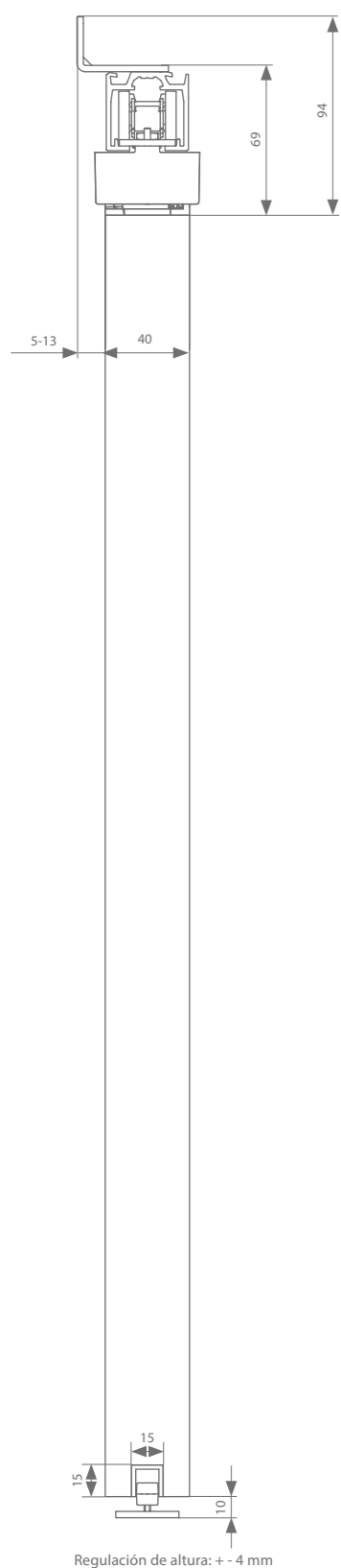
Fijación vista a pared 40 mm
