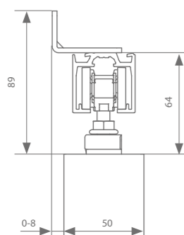
Fijación vista a pared 50 mm
