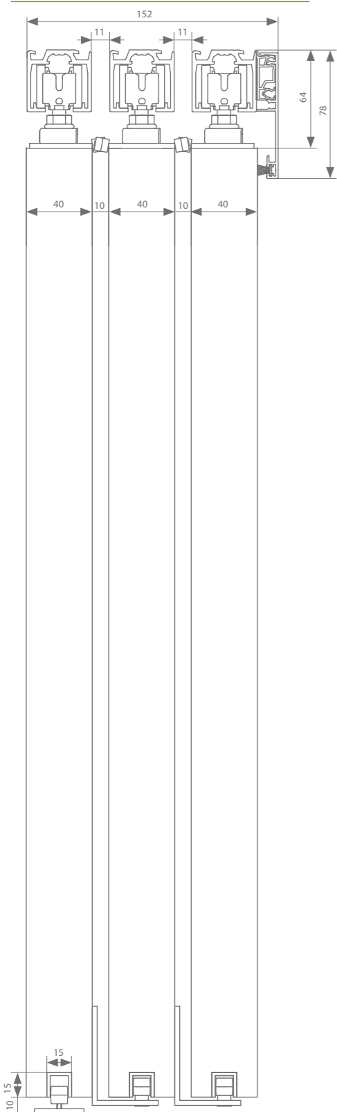
Paralelo fijación vista a techo 1
