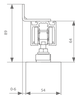
Fijación vista a pared 54 mm
