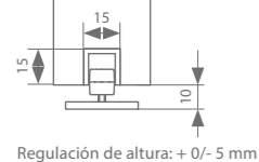
Regulación de altura: + 0/- 5 mm
