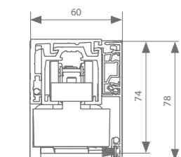
Fijación vista a pared 40 mm
