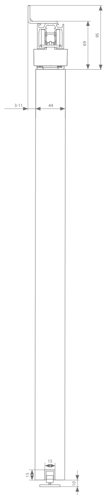
Fijación vista a pared 44 mm
