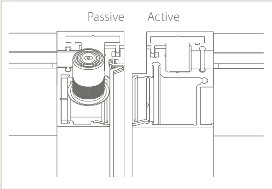
Encadrement de sol et encadrement de plafond de la porte battante double Divina
