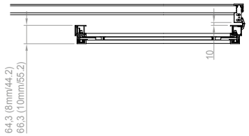
Porte battante simple Divina en position ouverte
