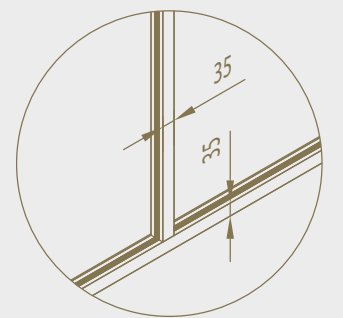
Profilés minimalististes de 35 mm de large convenant à différentes épaisseurs de verre
