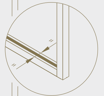
Finition identique des deux côtés
