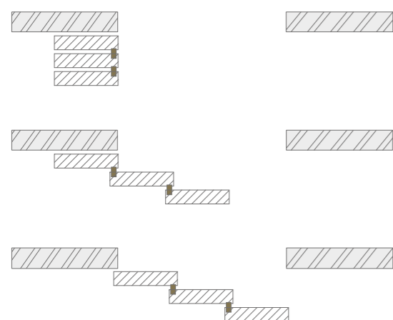
Version avec entraîneur
