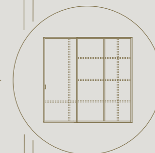
Optionele tussenregels met vrij te kiezen positie
