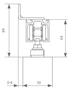
Muurbevestiging 50 mm
