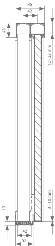
zonder bovengeleiding
