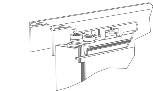
met bovengeleiding
