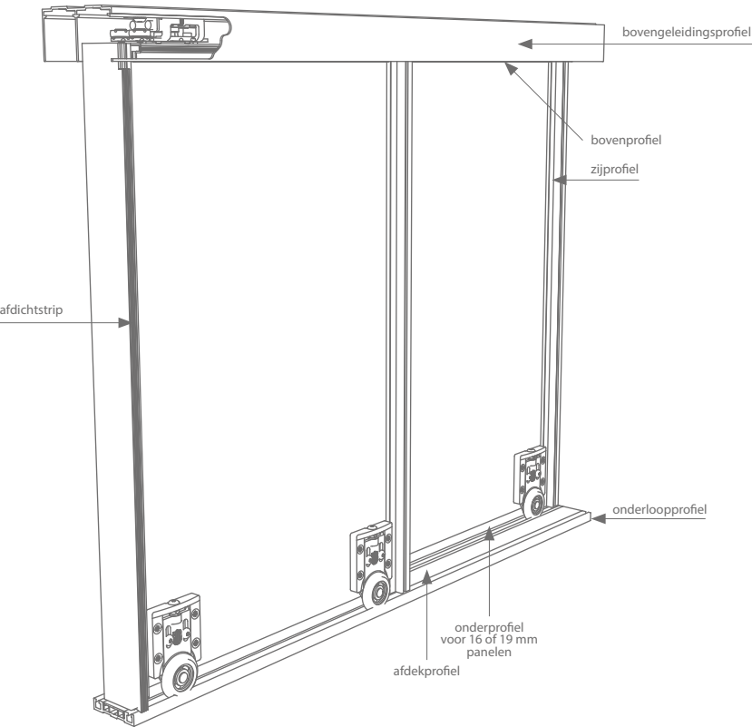
met bovengeleiding
