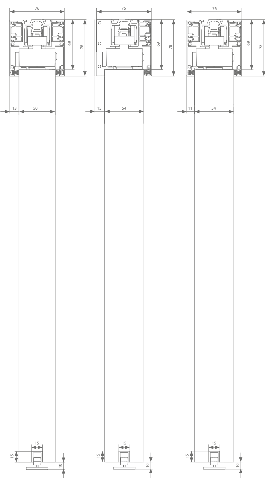
fixation au plafond 54 mm
