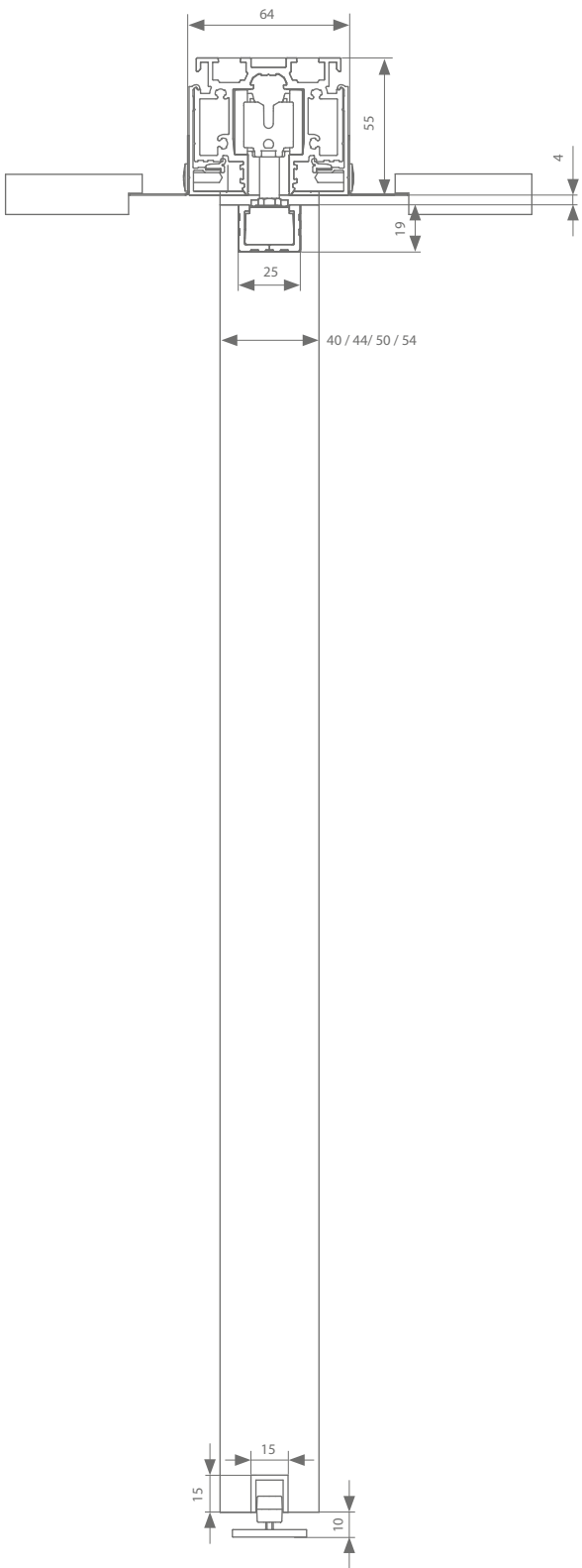
Pour plafond technique (1+2)
