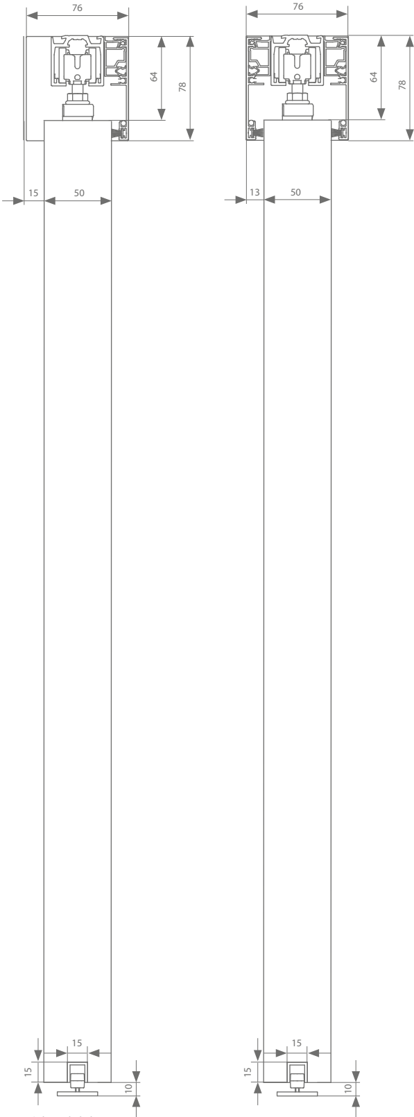
fixation au plafond 50 mm
