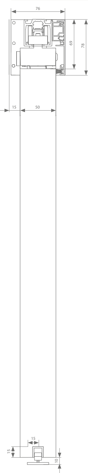
fixation au plafond 50 mm
