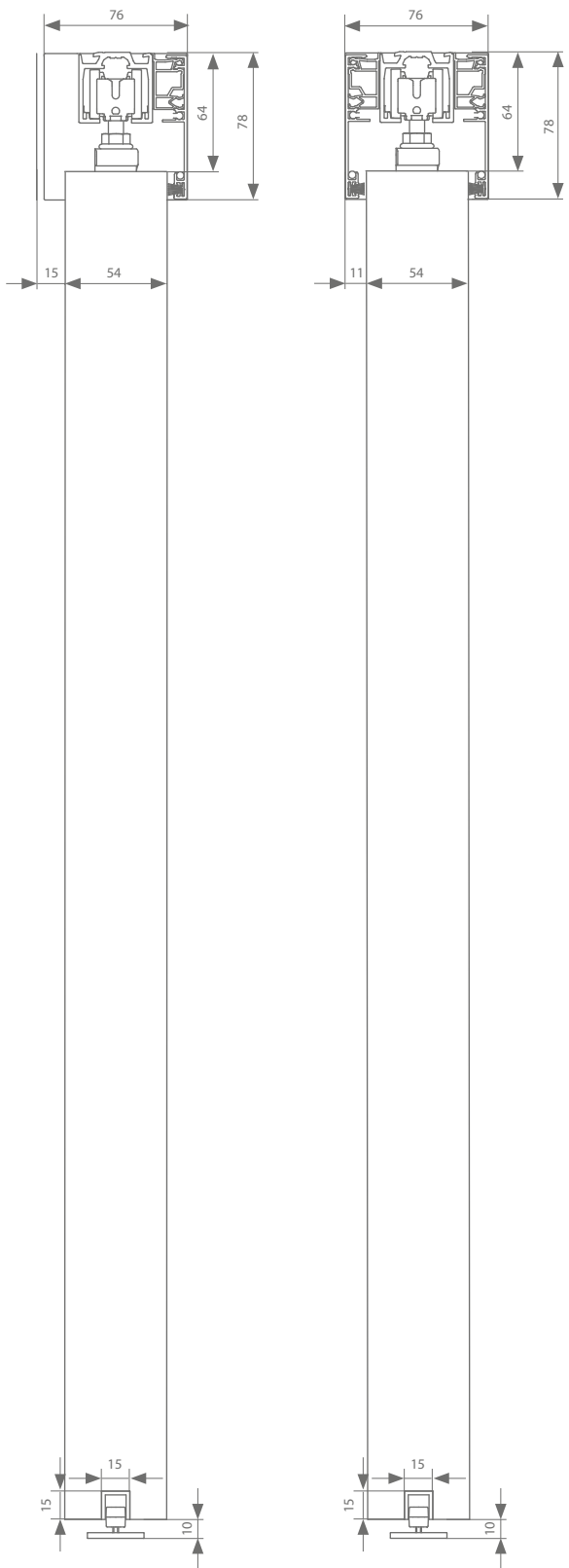
fixation au plafond 54 mm
