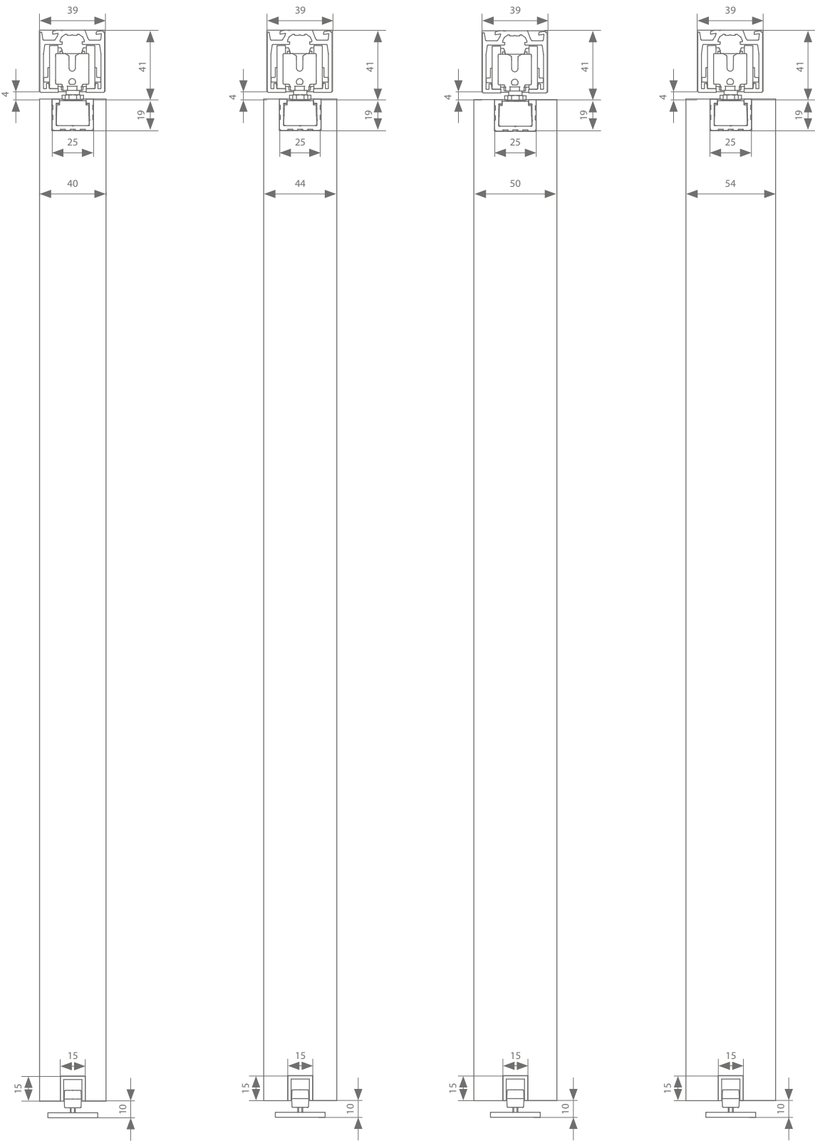
fixation au plafond 40 mm fixation au plafond 44 mm fixation au plafond 50 mm fixation au plafond 54 mm
