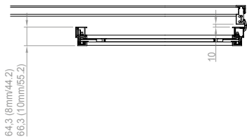
Divina Einzeltür, Schwingtür, geöffnete Position
