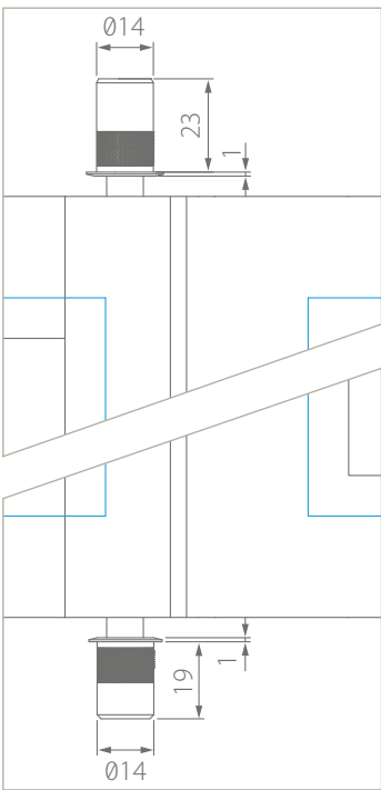
Vloerhuls en plafondhuls van divina dubbele draaideur
